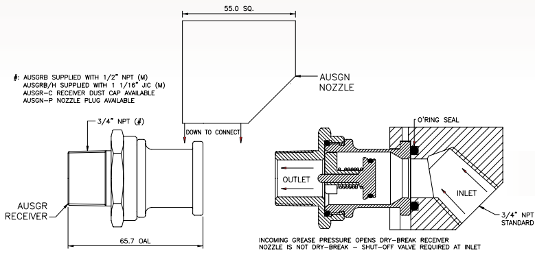
AUSGRC Receiver Cap AUSGR Receiver AUSGN Nozzle AUSGNP Nozzle Plug
